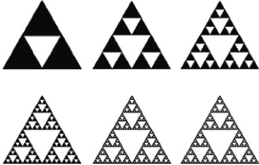
Şekil 5. 2. Sierpinski üçgeni.
